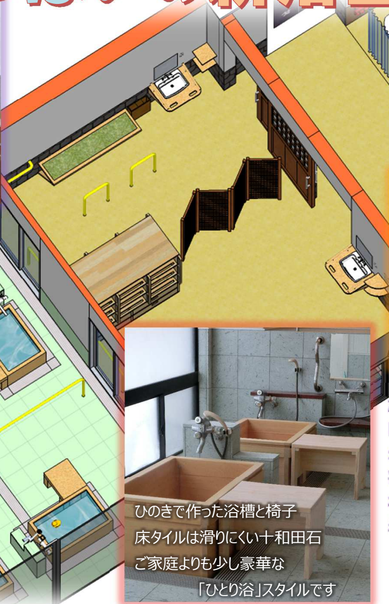
適所に手すりを配置し、安全で使い勝手の良い脱衣場
